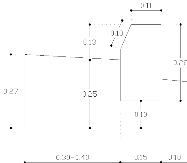
Λεπτομέρεια Κρασπεδόρειθρου
