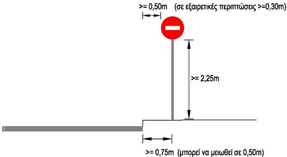
Σχήμα 5: Τοποθέτηση πινακίδας σε αστική οδό με πεζοδρόμιο
