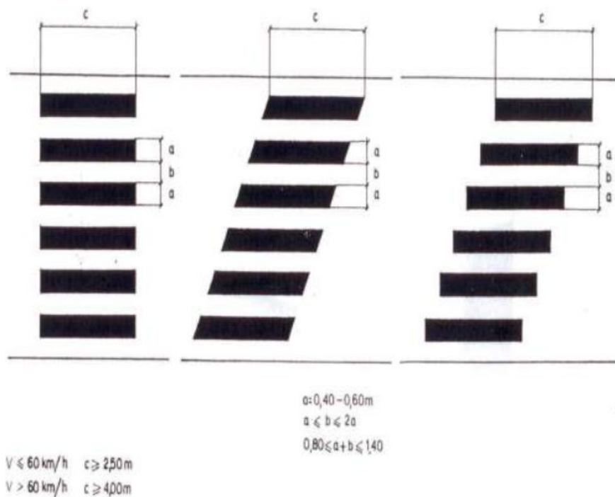
Σχήμα 6: Διαγράμμιση διαβάσεων πεζών
