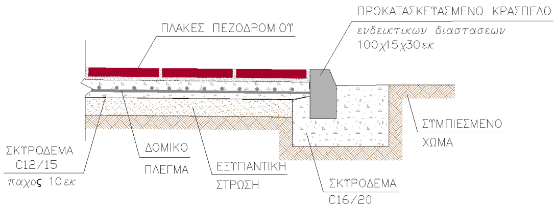
Σχήμα 1: Επίστρωση πεζοδρομίου με πλάκες από σκυρόδεμα
