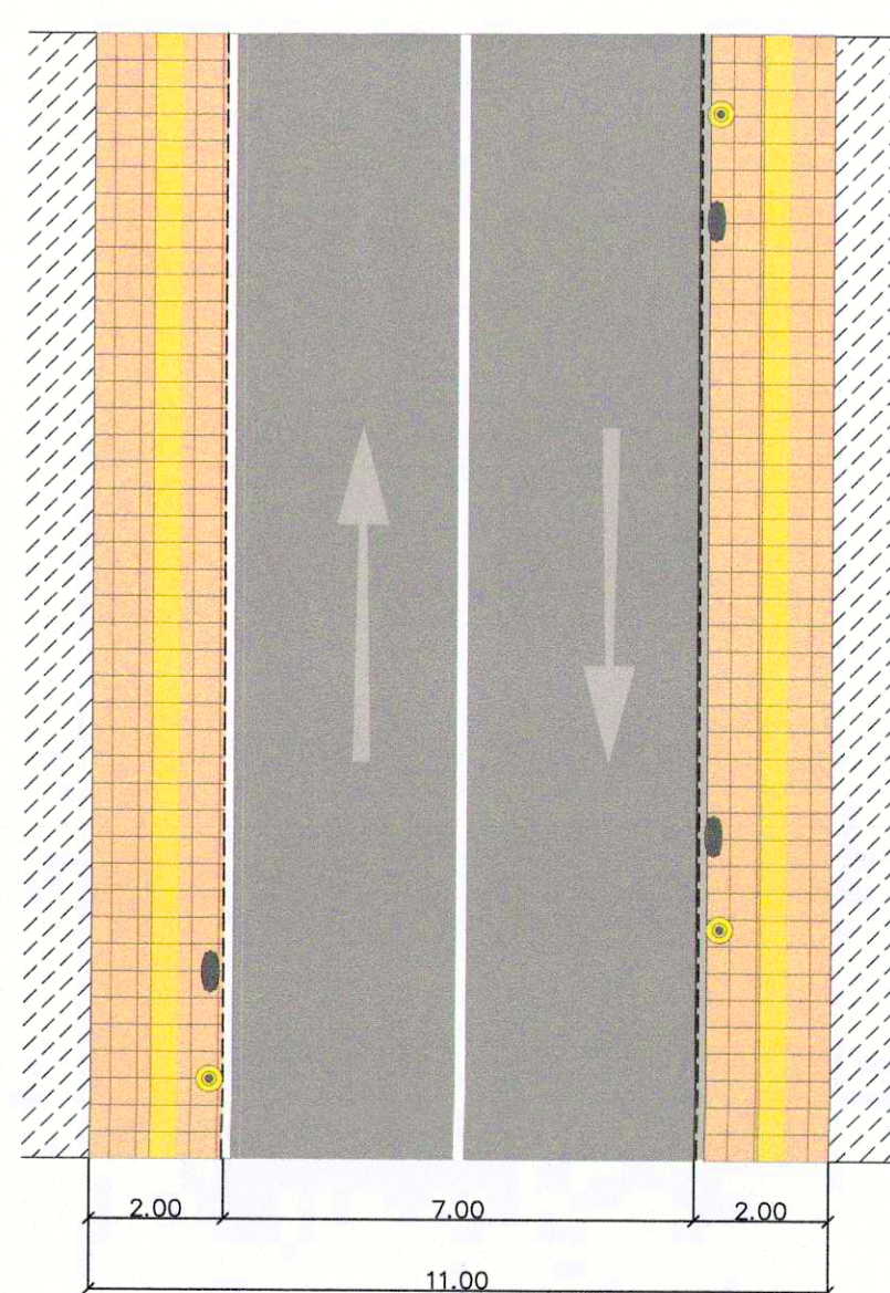
ΤΥΠΙΚΗ ΔΙΑΤΟΜΗ
