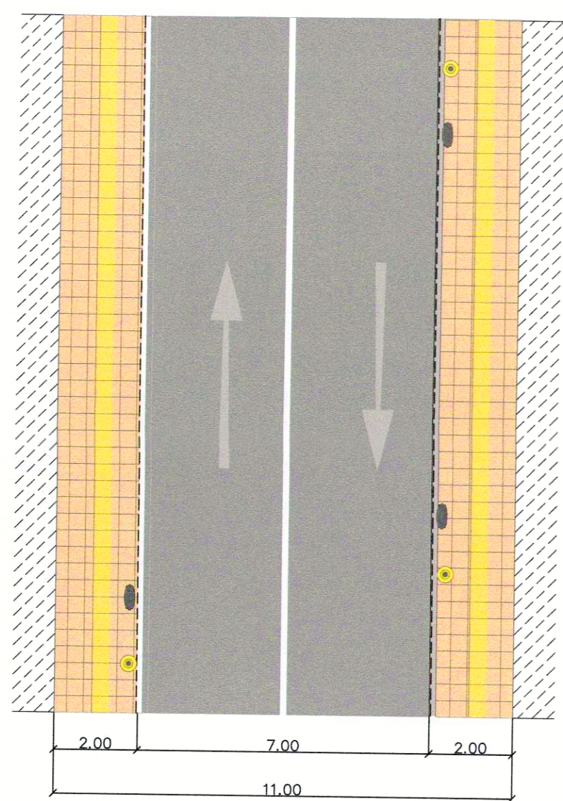
ΤΥΠΙΚΗ ΔΙΑΤΟΜΗ
