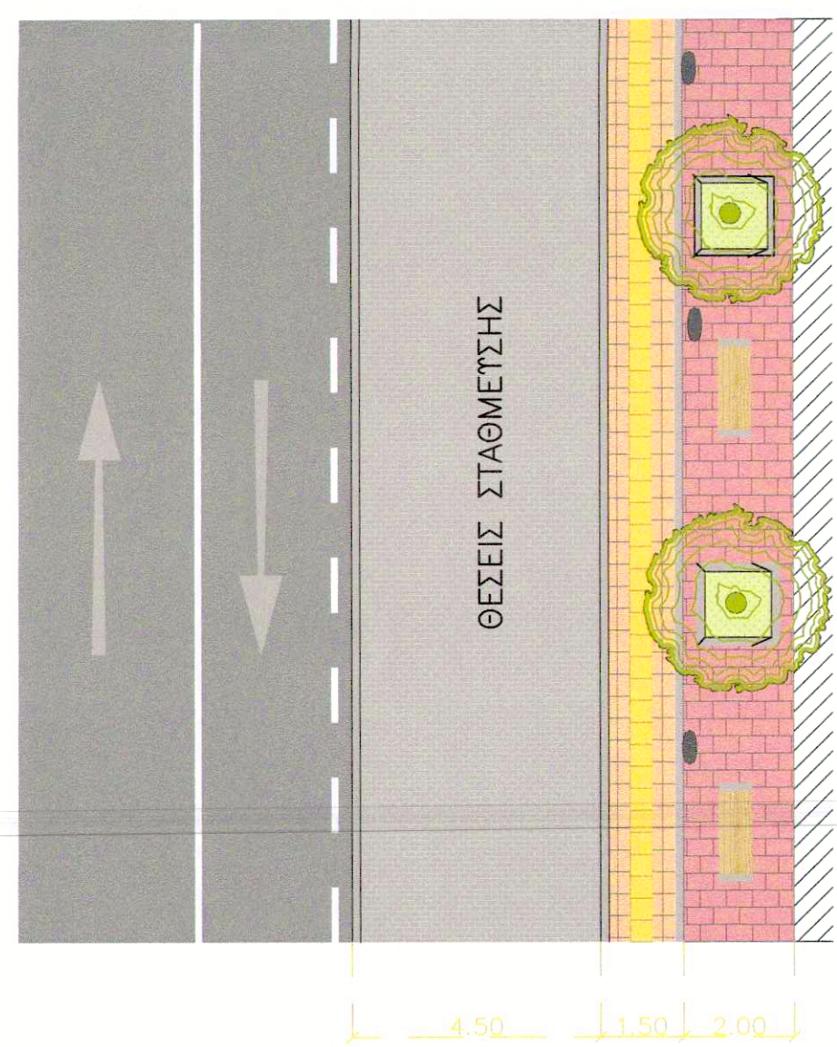
ΤΥΠΙΚΗ ΔΙΑΤΟΜΗ 2 (ΓΗΠΕΔΟ) ΟΔΟΥ Λ. ΔΗΜΟΚΡΑΤΙΑΣ
