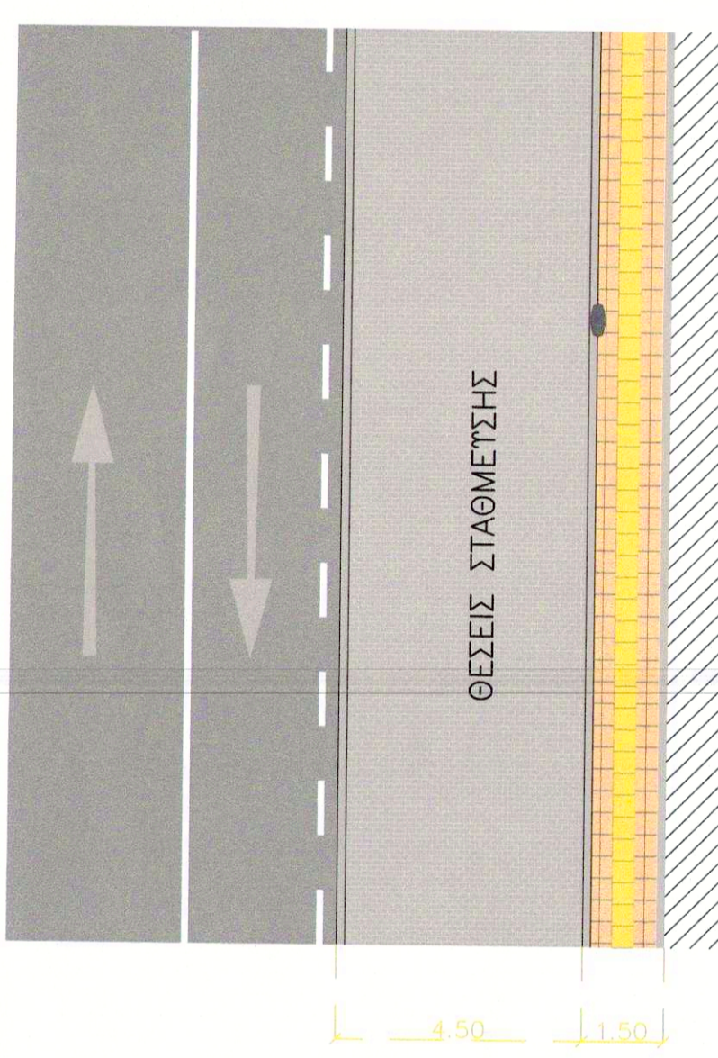
ΤΥΠΙΚΗ ΔΙΑΤΟΜΗ 3 (ΝΕΚΡΟΤΑΦΕΙΟ) ΟΔΟΥ Λ. ΔΗΜΟΚΡΑΤΙΑΣ
