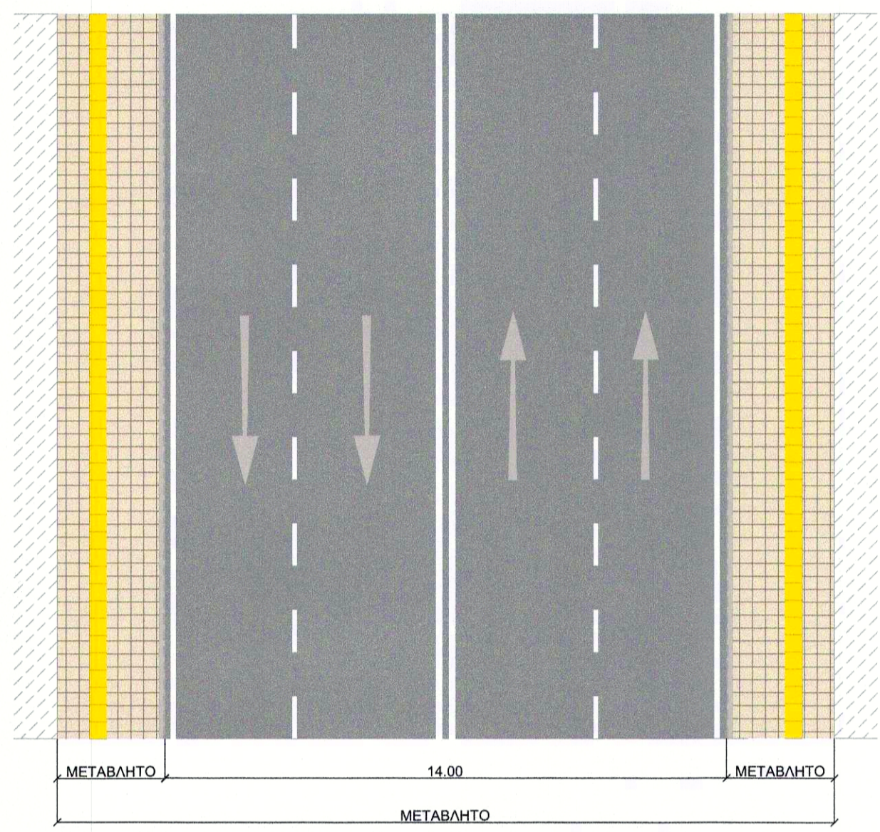
ΤΥΠΙΚΗ ΔΙΑΤΟΜΗ
