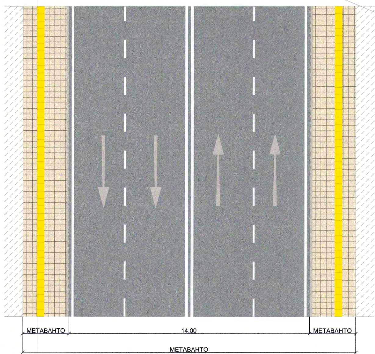
ΤΥΠΙΚΗ ΔΙΑΤΟΜΗ
