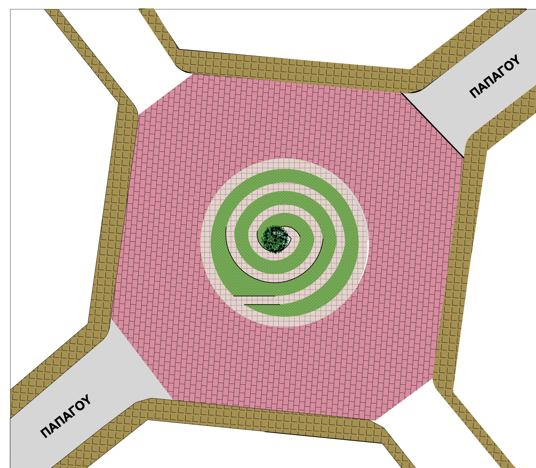
ΚΥΚΛΙΚΟΣ ΚΟΜΒΟΣ ΣΤΡ. ΠΑΠΑΓΟΥ
