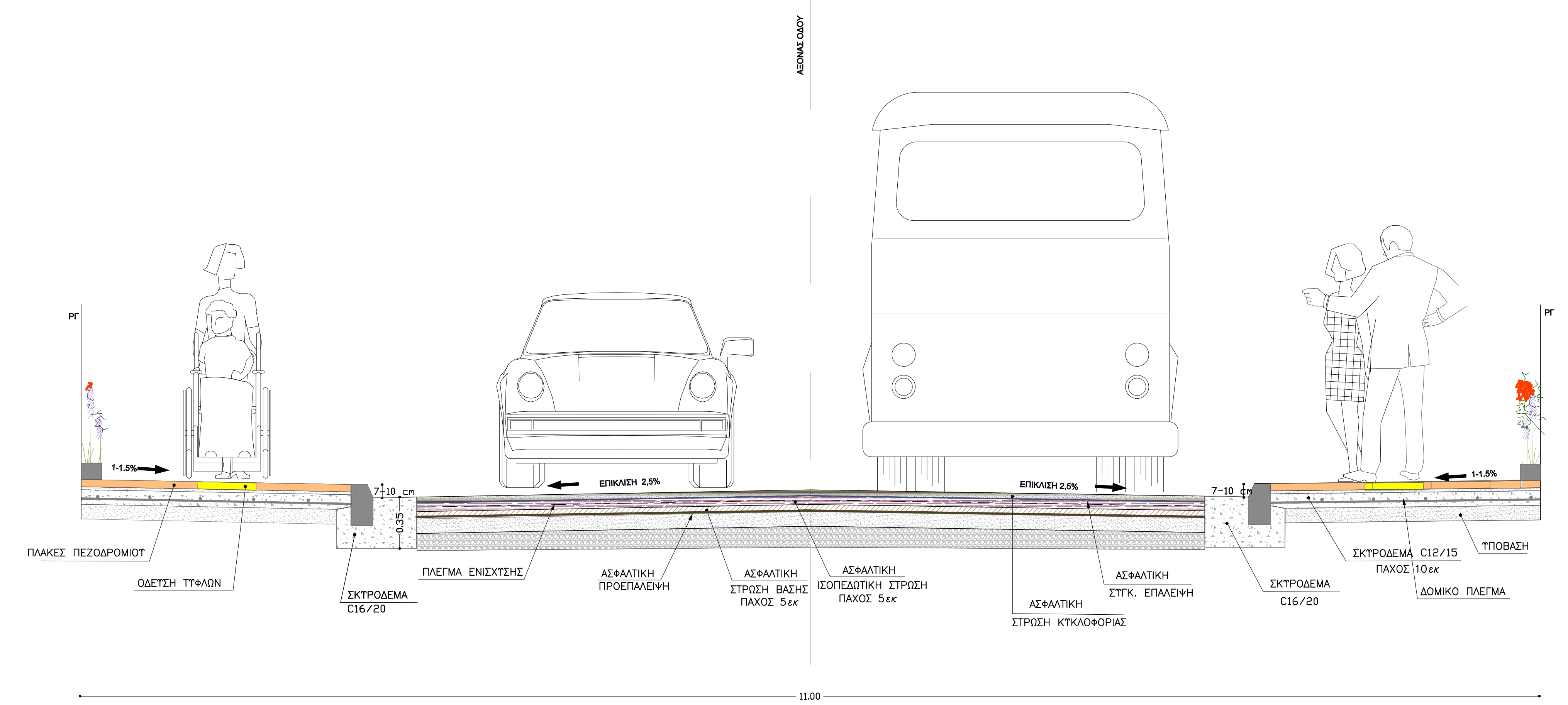
ΤΟΜΗ Α-Α ΚΛΙΜΑΚΑ 1:20
