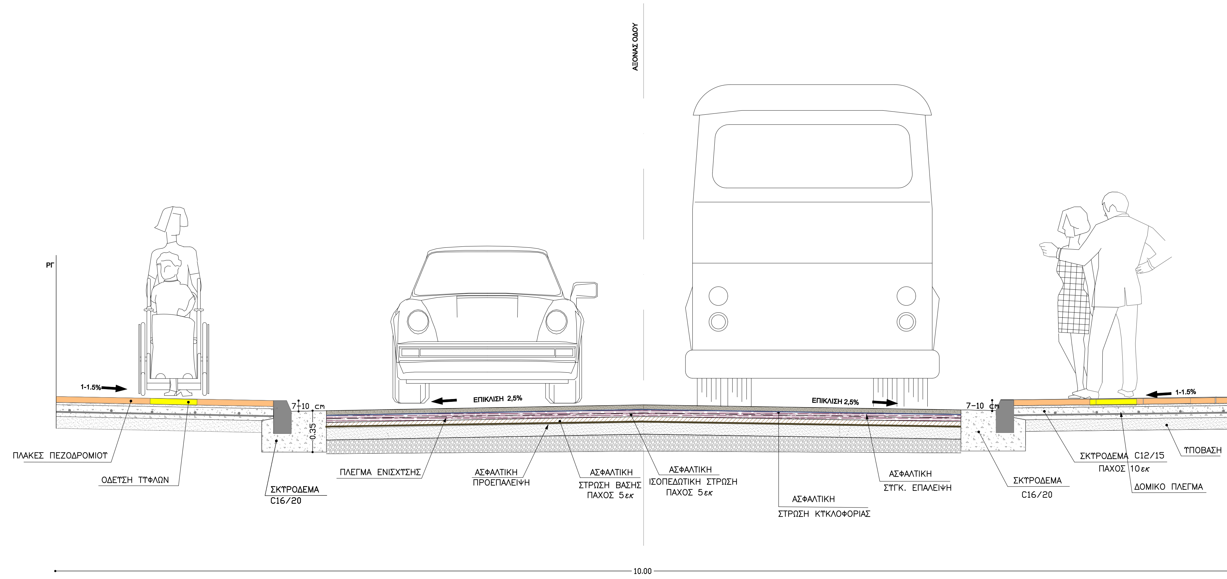
ΤΟΜΗ Α-Α ΚΛΙΜΑΚΑ 1:20
